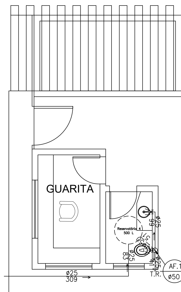
● ABASTECIMENTO DE ÁGUA FRIA ESC.: 1/50
