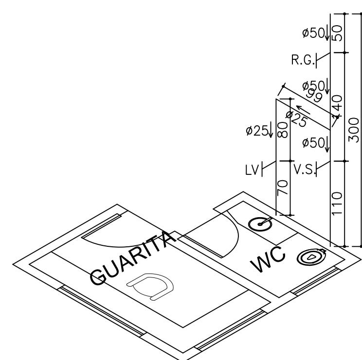
● ISOMÉTRICO ESC.: 1/50
