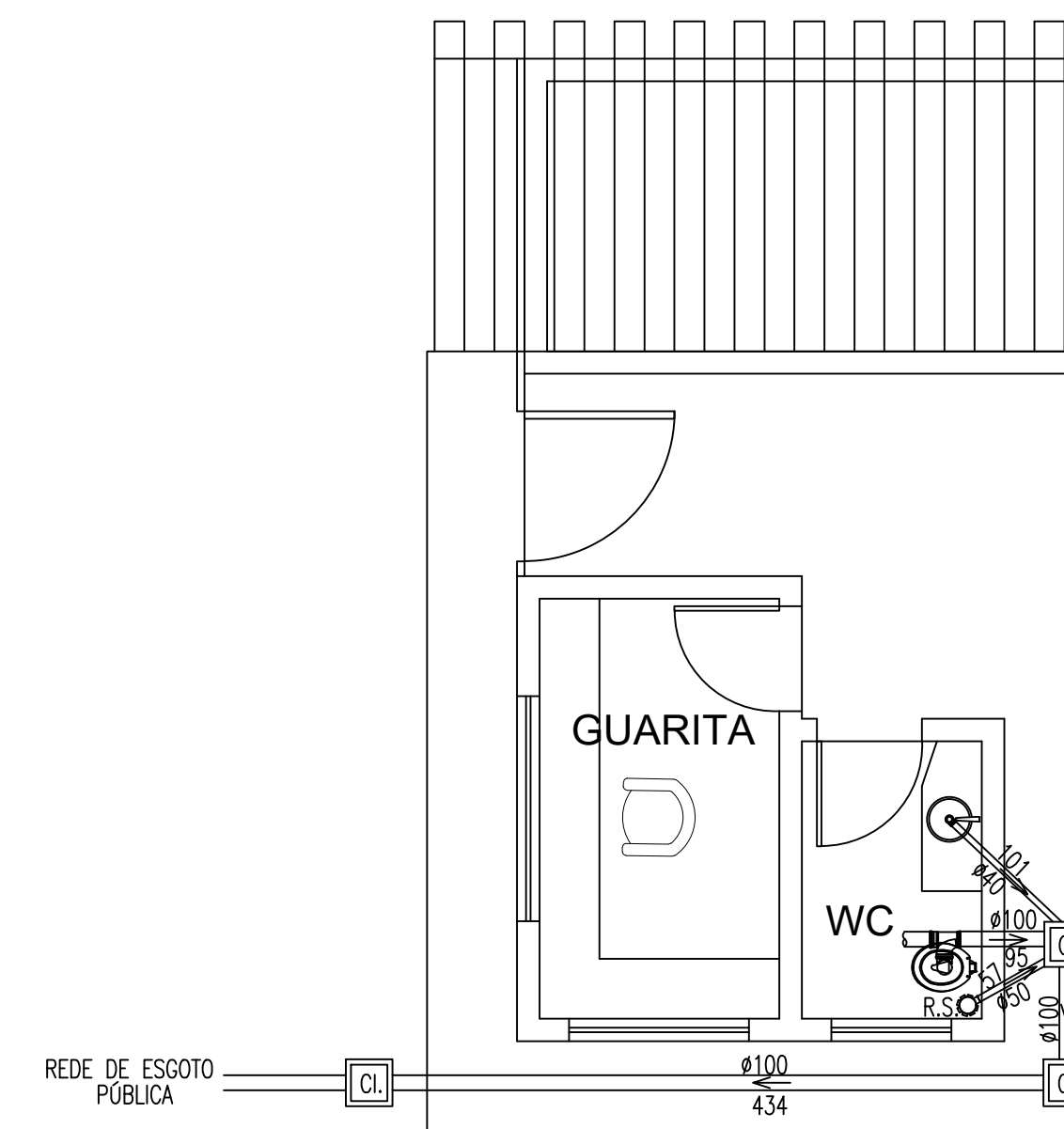
● REDE ESGOTO ESC.: 1/50
